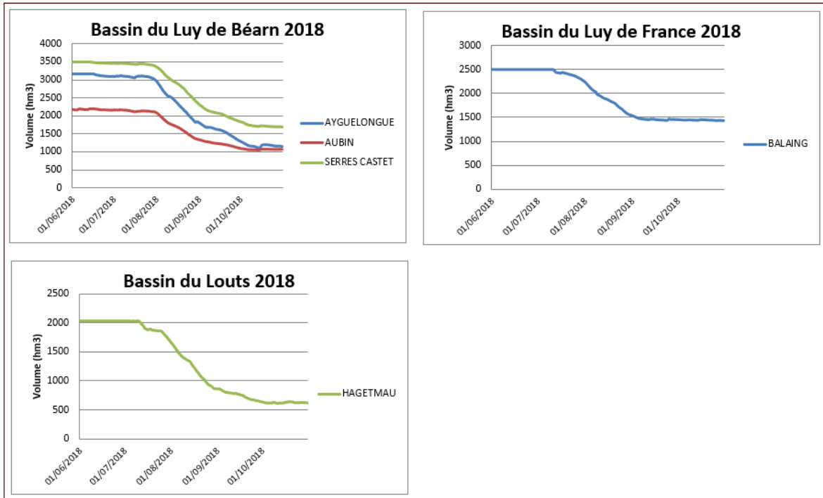
Figure 23 : Courbes de vidange des réservoirs pour l'été 2018
